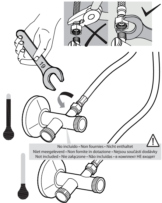
Blocaje superior • Système de blocage supérieur Oberes Verschlussystem • Bovenafsluiting Bloccaggio superiore • Horní blokáda Upper locking system • Blokada górna
