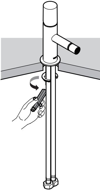
Blocaje superior • Système de blocage supérieur Oberes Verschlussystem • Bovenafsluiting Bloccaggio superiore • Horní blokáda Upper locking system • Blokada górna
